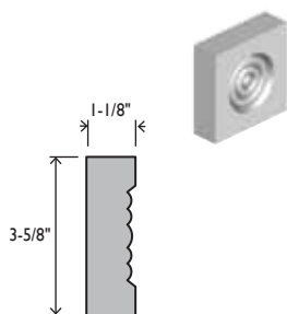
EC28 ROSETTE 1-1/8 X 3-5/8 X 3-5/8
