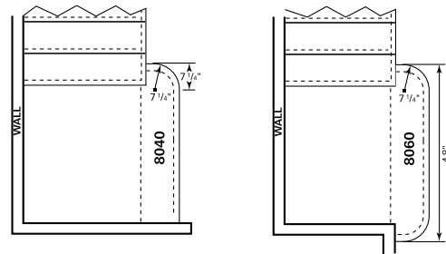
8040 / 8840 / 8940 - 48" & 60"
