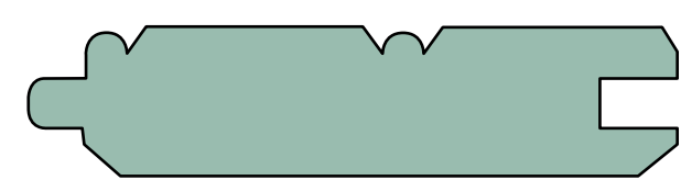
1 X 4 "C" EDGE & CENTERBEAD / V-JOINT
